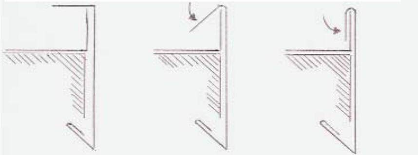
Stirnbrettverkleidung durch Rollenwechsel in 2 Arbeitsschritten (bei breiterem Einkantungen)
